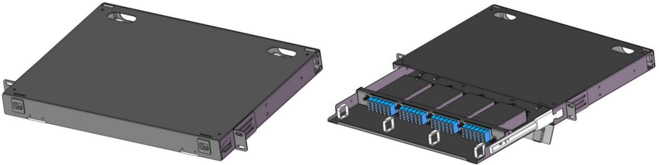
1Usize: 438mm (D) 334mm (W)
